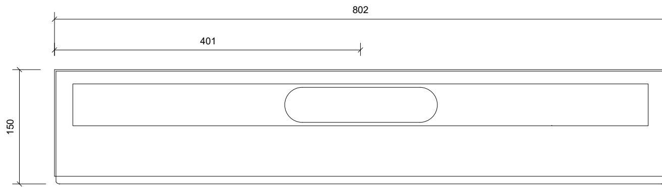
Plan/Plan/Draufsicht
