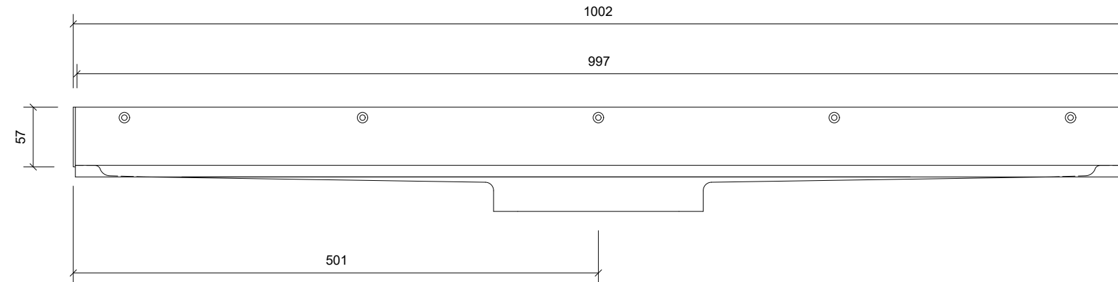
Front Opstalt/Front Elevation/Frontansicht
