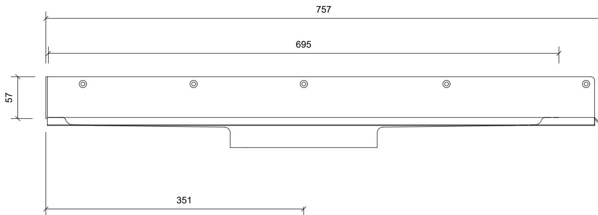
Front Opstalt/Front Elevation/Frontansicht
