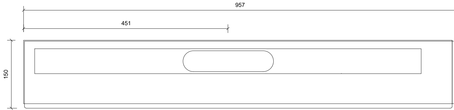
Plan/Plan/Draufsicht
