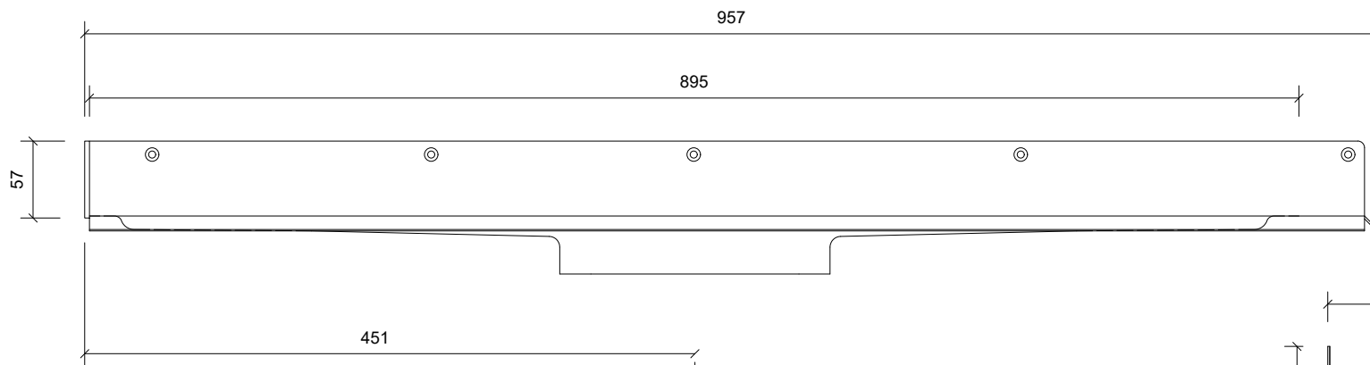
Plan/Plan/Draufsicht
