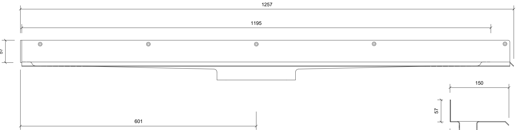
Front Opstalt/Front Elevation/Frontansicht
