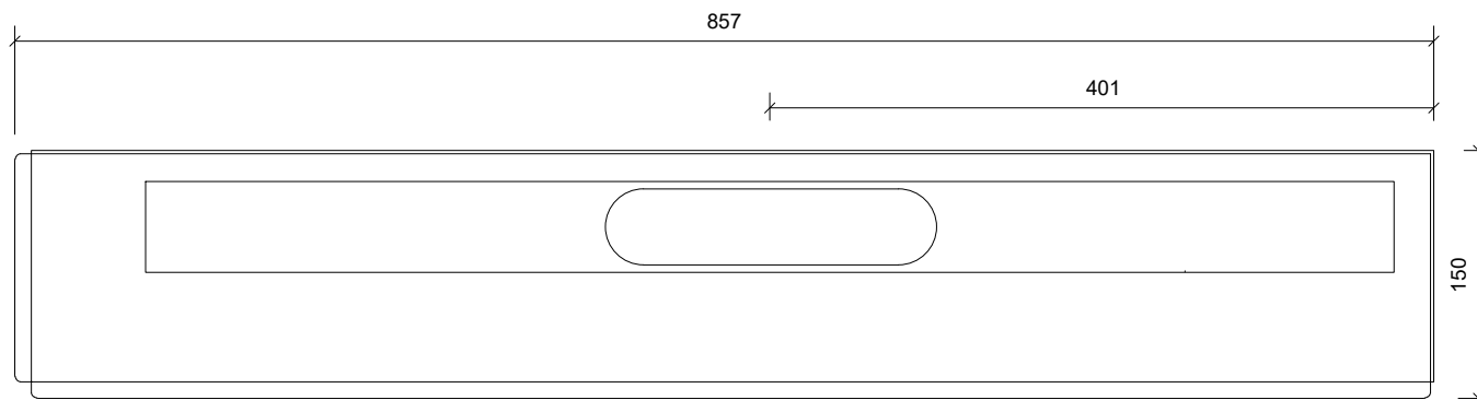
Plan/Plan/Draufsicht
