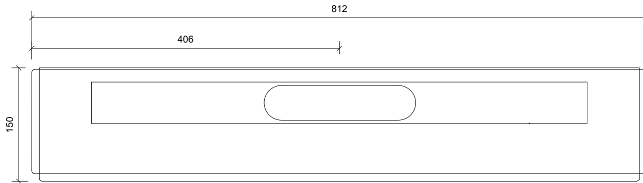
Plan/Plan/Draufsicht
