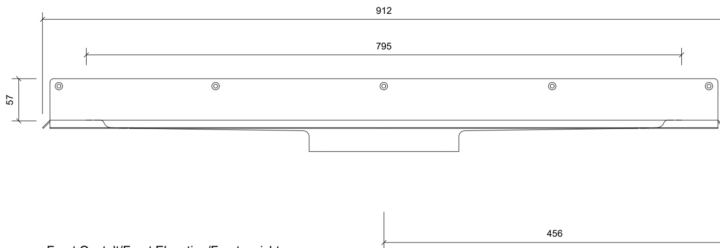
Front Opstal/Front Elevation/Frontansicht
