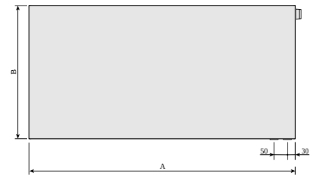
Plan Ventil Compact, set forfra til højre
