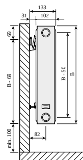
Compact type 22, set fra siden med Quick vægbeslag
