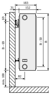
Compact type 33, set fra siden med Quick vægbeslag
