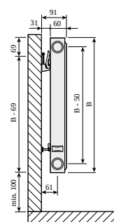
Compact type 11, set fra siden med Quick vægbeslag
