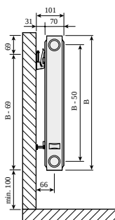
Compact type 21, set fra siden med Quick vægbeslag
