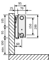
Plint, type 21s med Monclac vægbeslag, set fra siden
