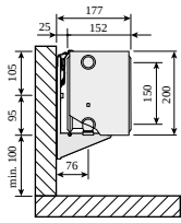
Plint, type 33 med Monclac vægbeslag, set fra siden
