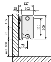
Plint, type 22 med Monclac vægbeslag, set fra siden
