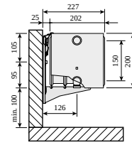
Plint, type 44 med Monclac vægbeslag, set fra siden
