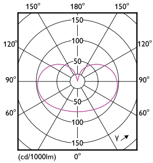
LEDlustre MAS P45 3,4W E27 927 FR-LDD
