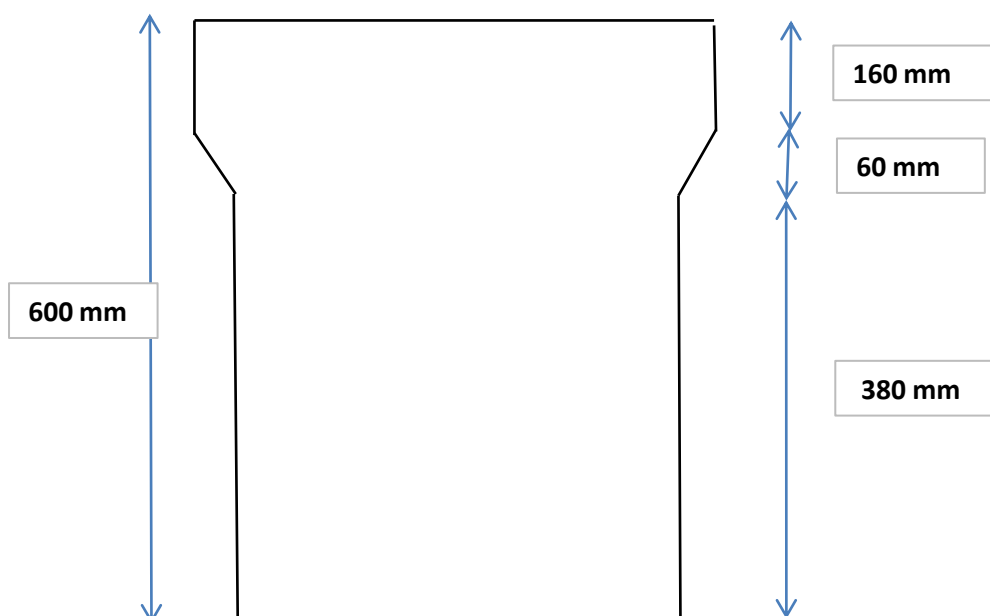
Justerbar Brøndskørt 425 mm
