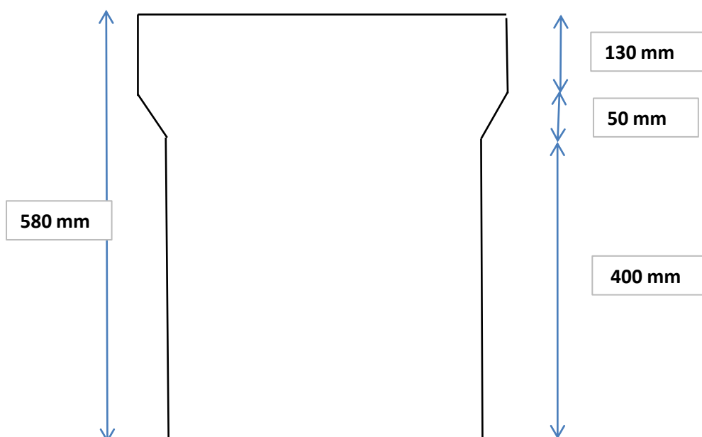
Justerbar Brøndskørt 600 mm
