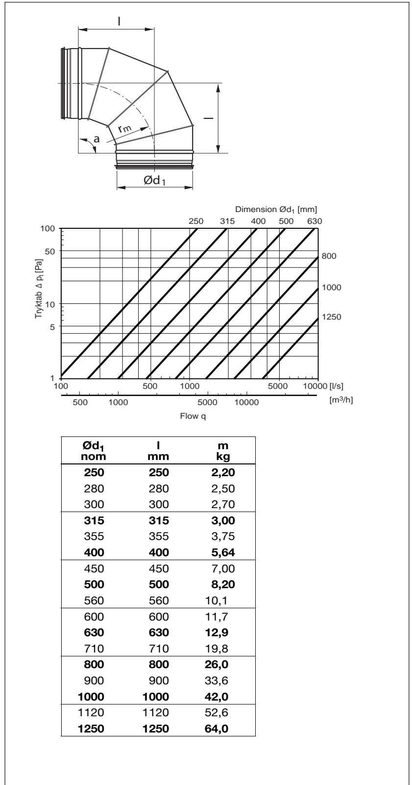
Falset bøjning samlet af segmenter. BFL-90 vises i eksemplet her til højre
