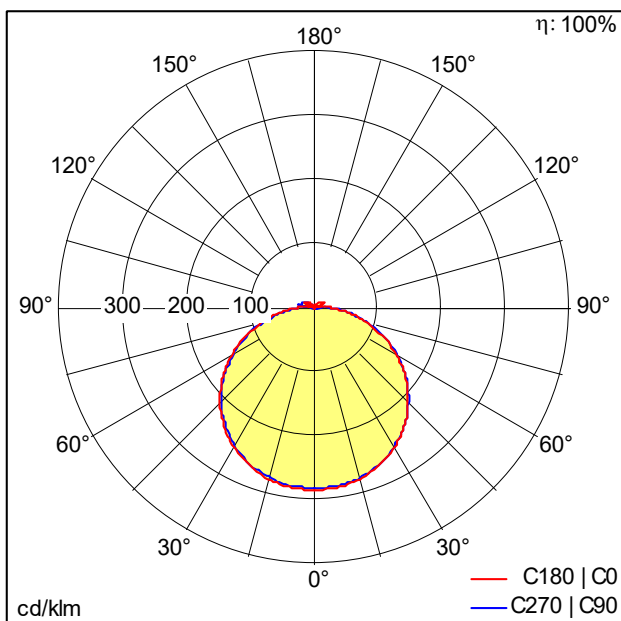
TE_LENA_VF_360_3500_840_FLEX1.ldt
