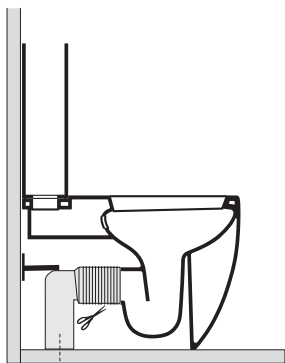
SW 90° 329004 max 160 min 70
