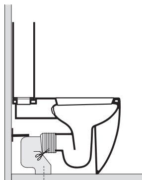
SW 329001 max 170 min 100
