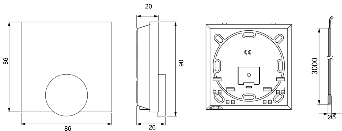
Figur 1: Dimensioner for analog COMFORT rumtermostat og ekstern føler (i mm)
