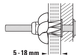
PowerKnot Rød Pan PT monteret i enkeltgips
