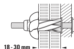
PowerKnot Sort COT med afstandsstykke - for montage af reolskinne
