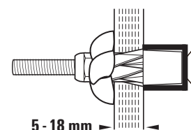
PowerKnot Rød COT med afstandsstykke - for montage af reolskinne
