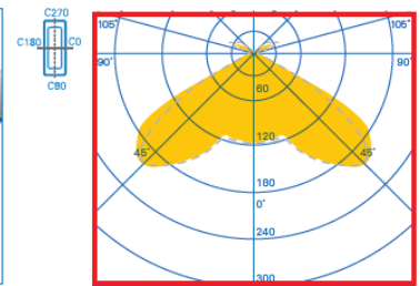
RoundTech MR Flugtvejebelysning - lysdistribution
