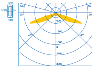
RoundTech MR Flugtvejebelysning - lysdistribution
