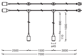
END DEC PEND7M 3X4W820 PLUG E27GY
