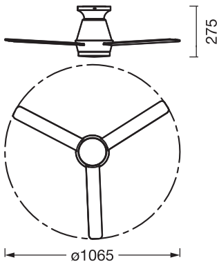
CEILING FAN NORDES 1065 38W CCTRGB
