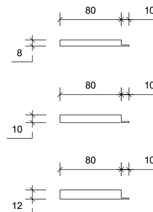
Side Opstalt/Side Elevation/Seitenansicht
