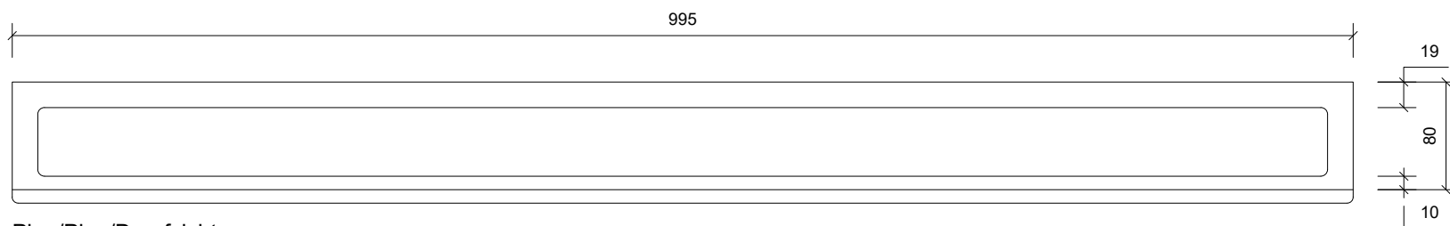
Plan/Plan/Draufsicht
