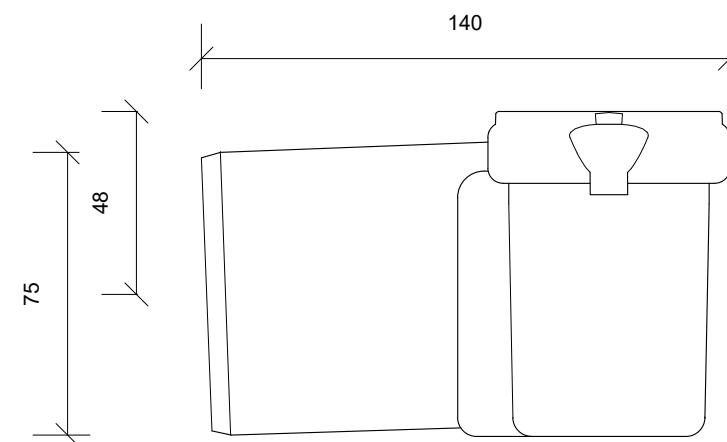
Side Opstalt/Side Elevation/Seitenansicht
