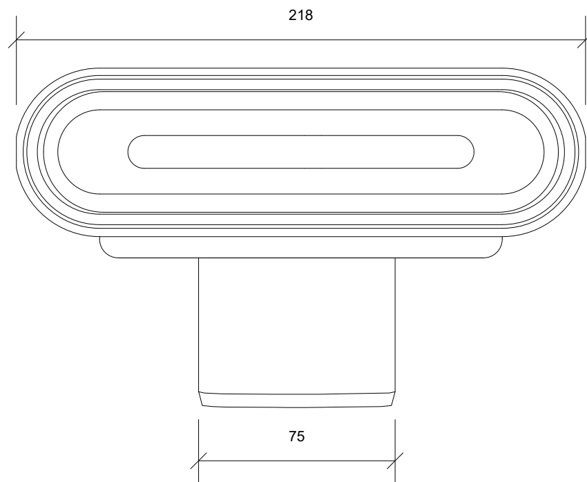
Plan/Plan/Draufsicht
