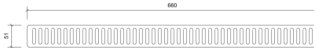
Plan/Plan/Draufsicht
