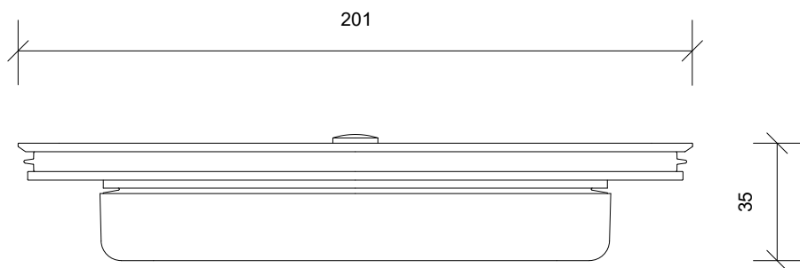
Front Opstalt/Front Elevation/Frontansicht
