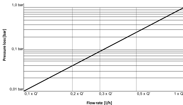
Typische Druckverlustkurve
