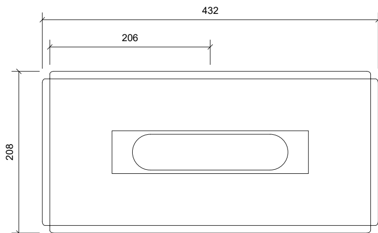
Plan/Plan/Draufsicht
