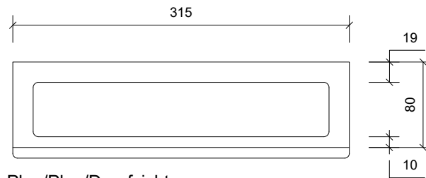
Plan/Plan/Draufsicht
