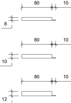
Side Opstalt/Side Elevation/Seitenansicht
