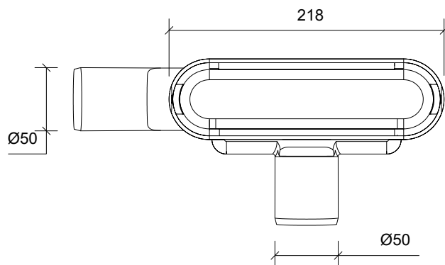
Plan/Plan/Draufsicht
