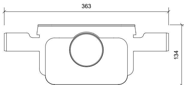
Front Opstalt/Front Elevation/Frontansicht
