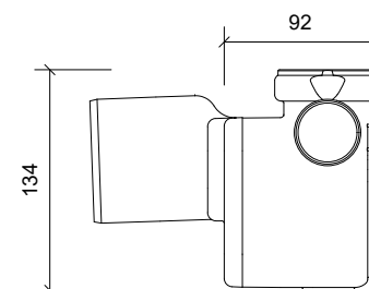
Side Opstalt/Side Elevation/Seitenansicht
