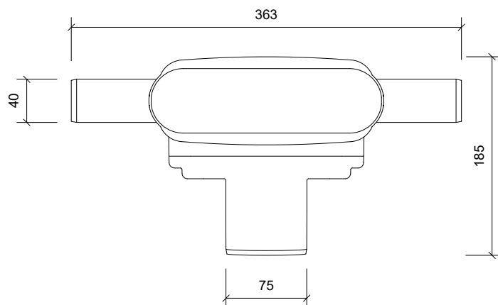
Plan/Plan/Draufsicht
