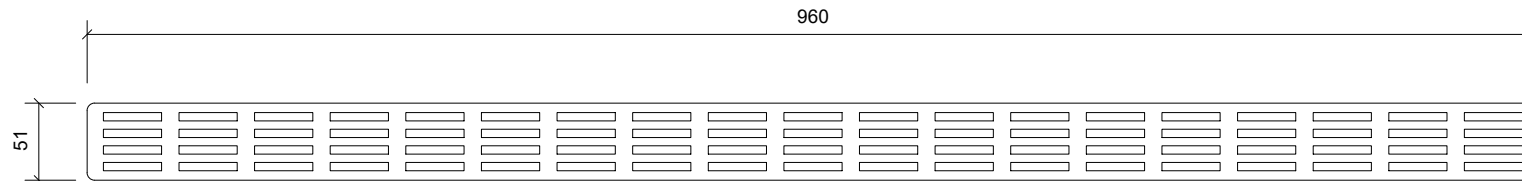
Plan/Plan/Draufsicht
