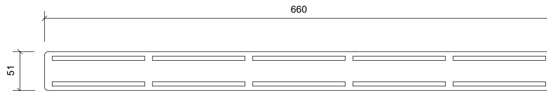
Plan/Plan/Draufsicht
