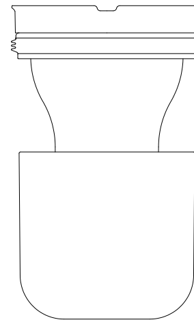
Side Opstalt/Side Elevation/Seitenansicht
