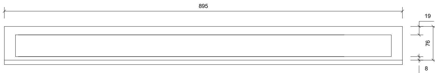
Plan/Plan/Draufsicht
