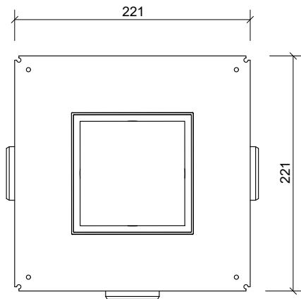
Plan/Plan/Draufsicht
