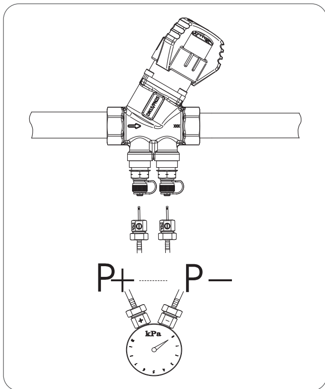
Måling af differensstryk ( \Delta p ) over ventilen
