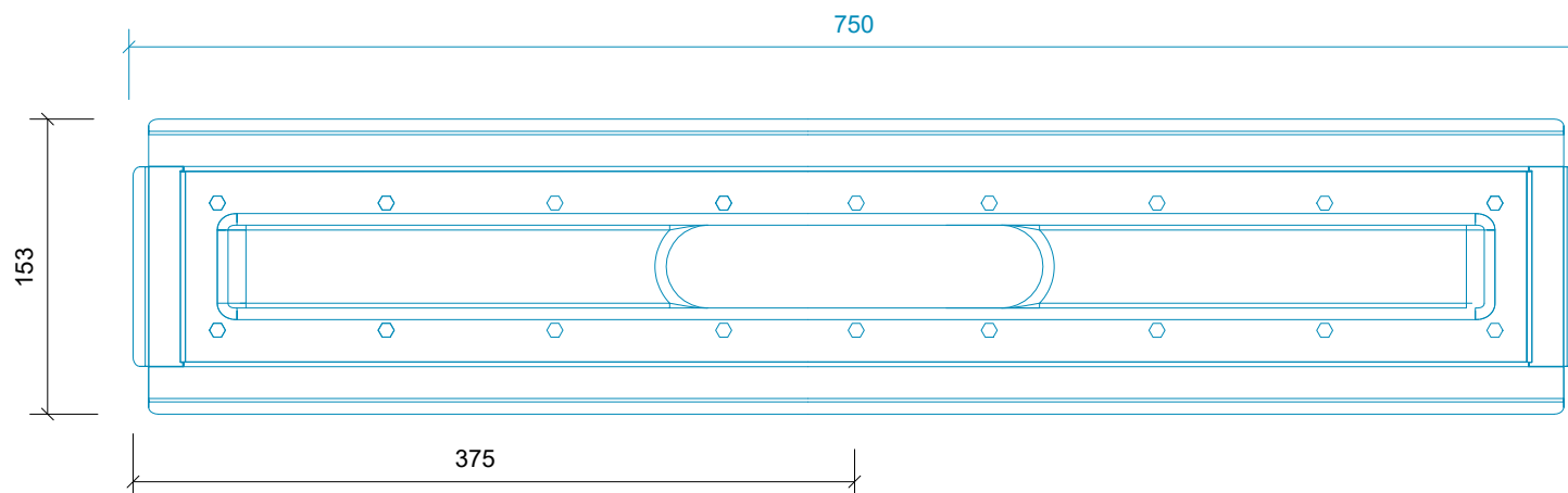
Plan/Plan/Draufsicht
