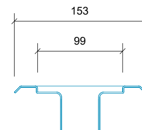
Side Opstalt/Side Elevation/Seitenansicht
