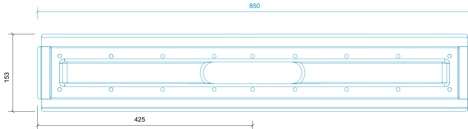
Plan/Plan/Draufsicht
