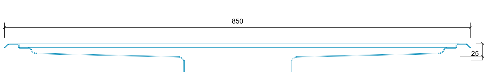
Front Opstalt/Front Elevation/Frontansicht
