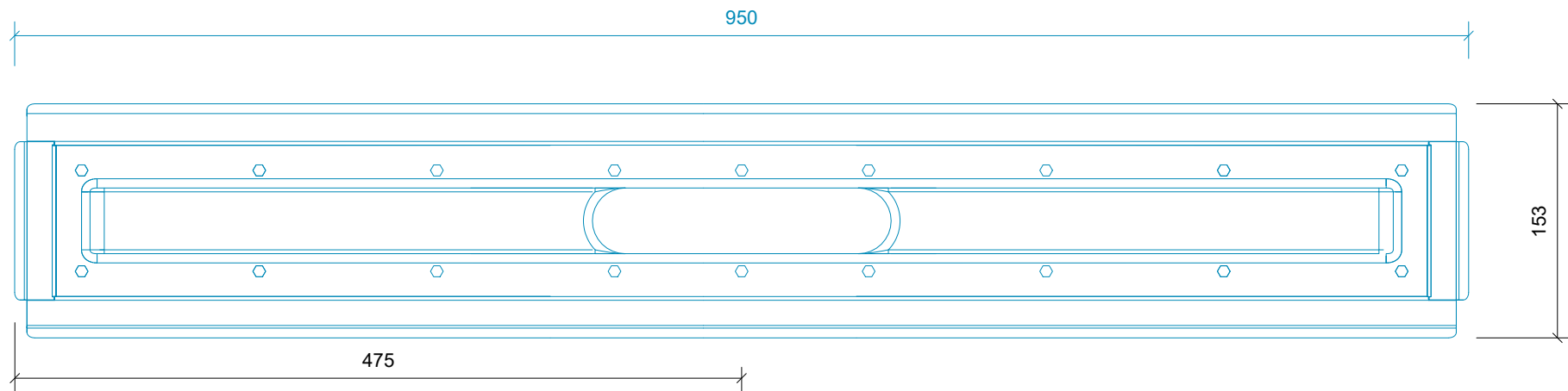
Plan/Plan/Draufsicht
