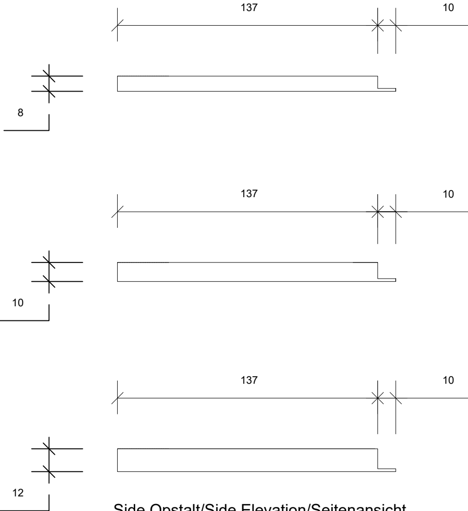
Side Opstalt/Side Elevation/Seitenansicht
