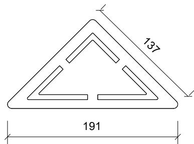
Plan/Plan/Draufsicht
