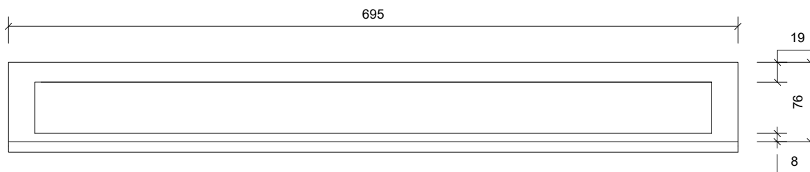
Plan/Plan/Draufsicht
