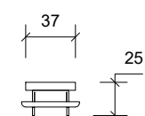
Side Opstalt/Side Elevation/Seitenansicht
