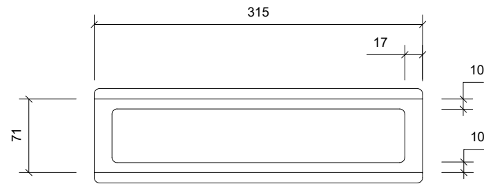
Plan/Plan/Draufsicht
