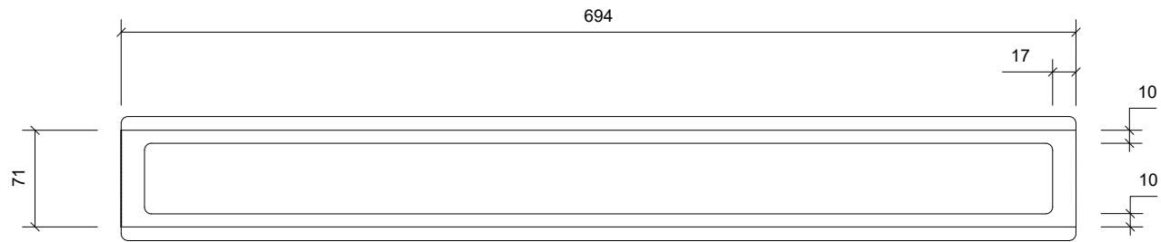
Plan/Plan/Draufsicht
