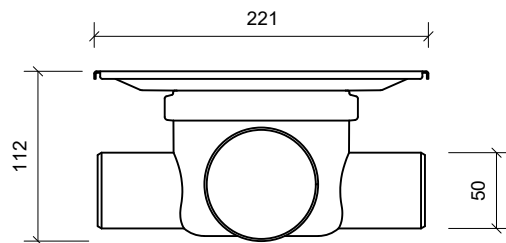
Front Opstalt/Front Elevation/Frontansicht
