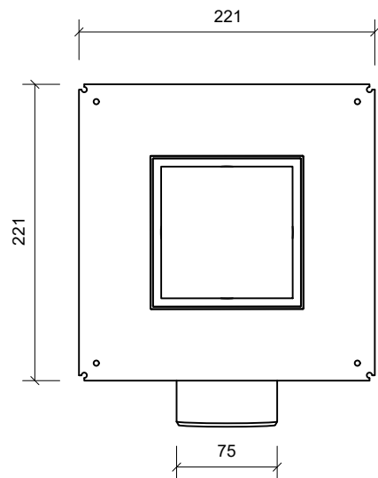
Plan/Plan/Draufsicht
