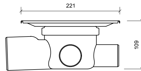
Side Opstalt/Side Elevation/Seitenansicht
