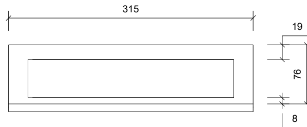
Plan/Plan/Draufsicht
