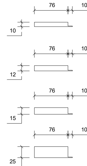
Side Opstalt/Side Elevation/Seitenansicht
